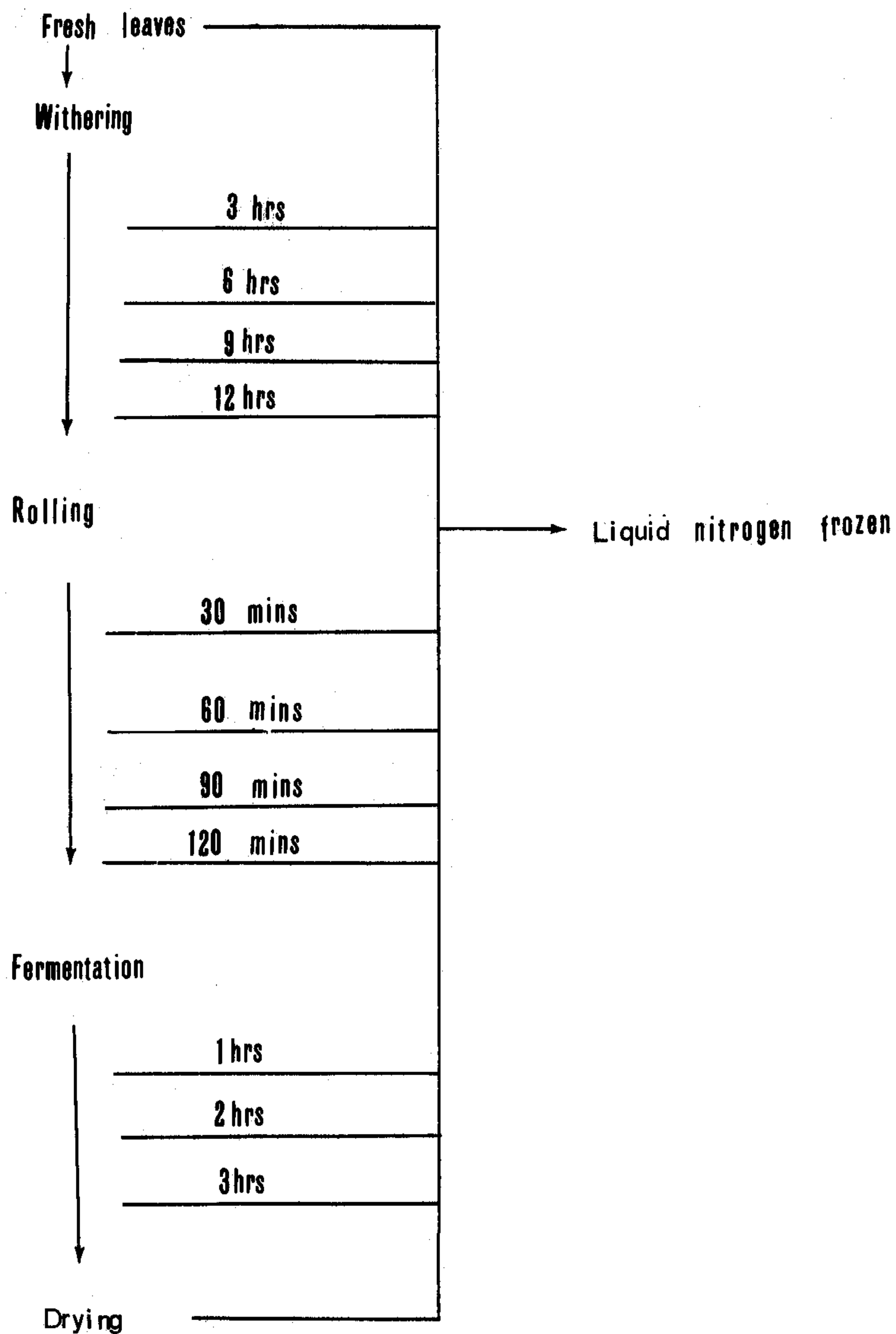
圖 2. 紅茶試樣製備流程圖
